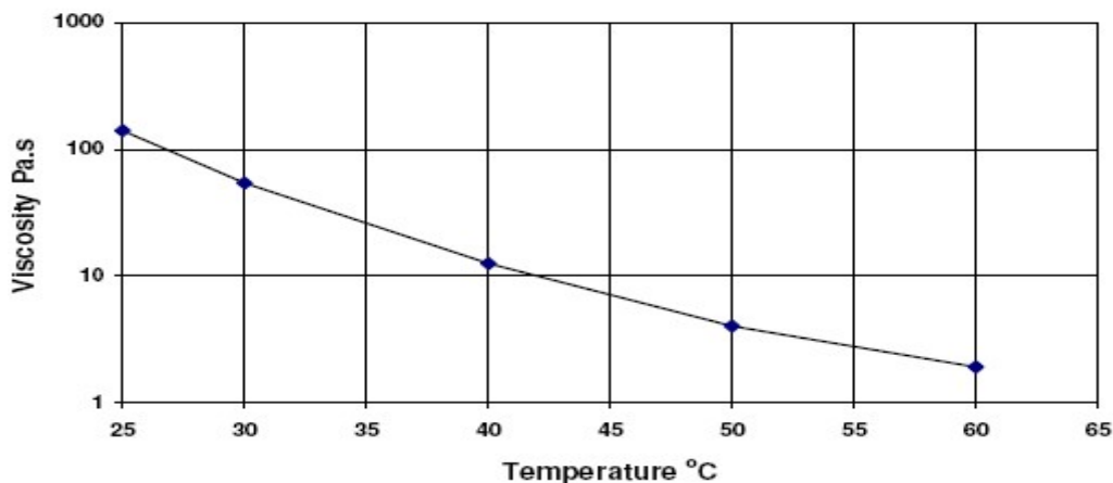
Cambios de la viscosidad con la Temperatura
